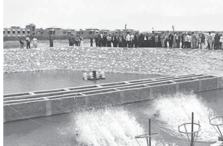
أحواض ترسيب مياه الصرف
